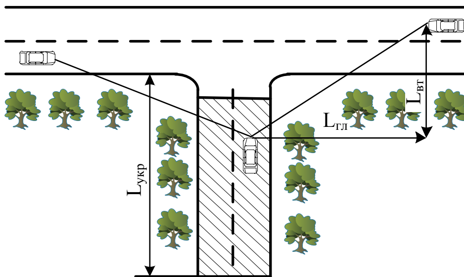
Рис. 2 – Схема для определения видимости на пересечении на одном уровне:
