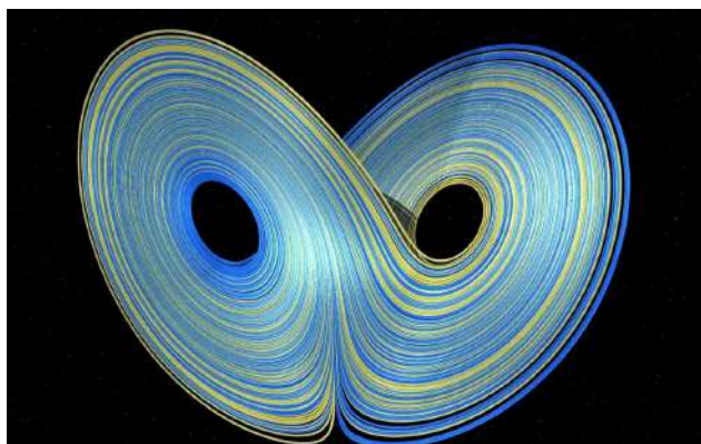
Рис. 5 – Странный аттрактор
