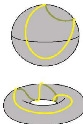
Рис. 4 – Стягивание петли
