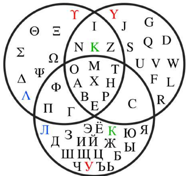
Рис. 2 – Сочетание множеств
