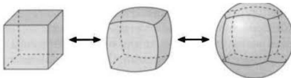
Рис. 3 – Гомеоморфизм сферы
